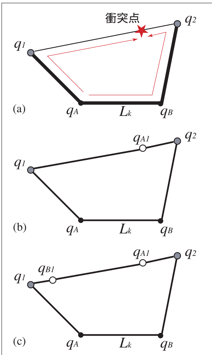
図 1: 衝突点ノードの挿入
