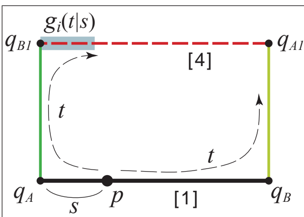
図 7: 軌跡リンク (グループ 1) の場合
