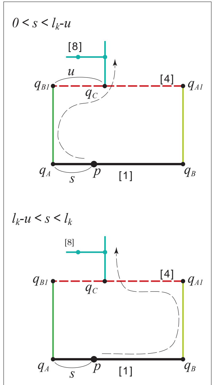
図 9: 軌跡リンク (グループ 1) 上に根を持つリンクの場合
