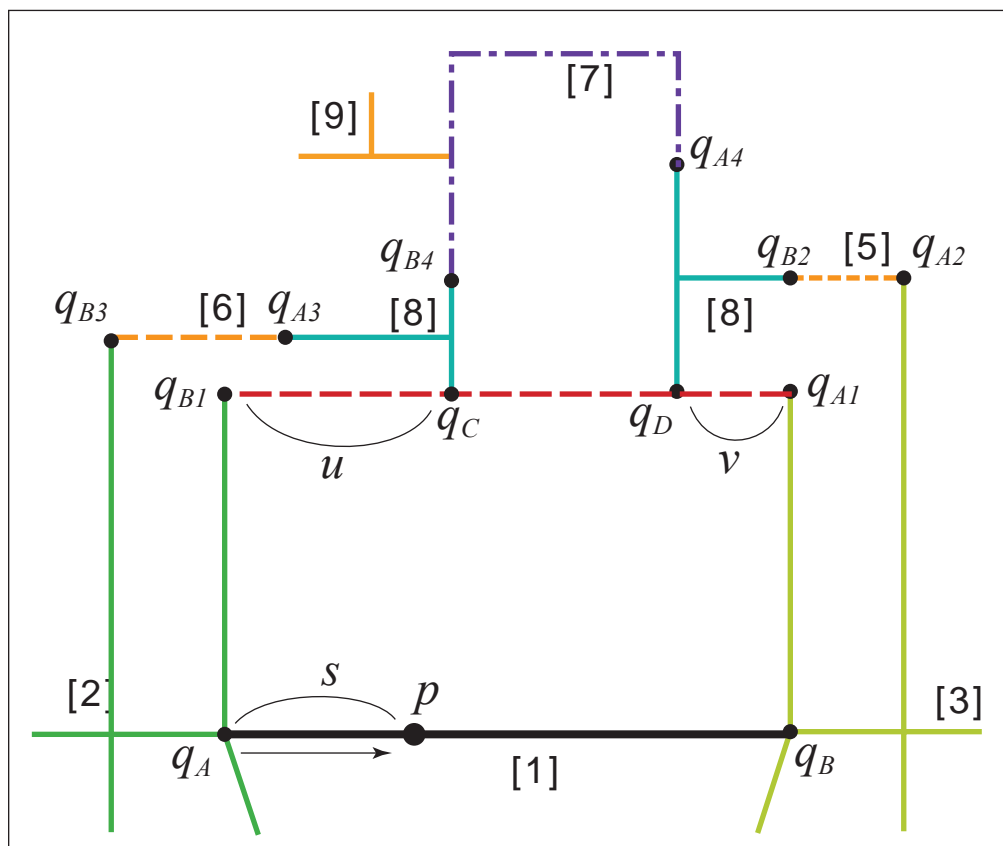
図 3: リンクの種類
