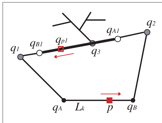
図 2: q_{p1} の軌跡リンク
