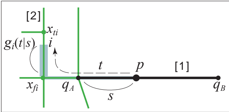
図 5: q_A からの最短経路が q_B を通らないリンクの場合
