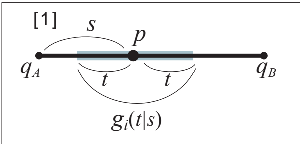
図 4: p の移動するリンク L_k の場合
