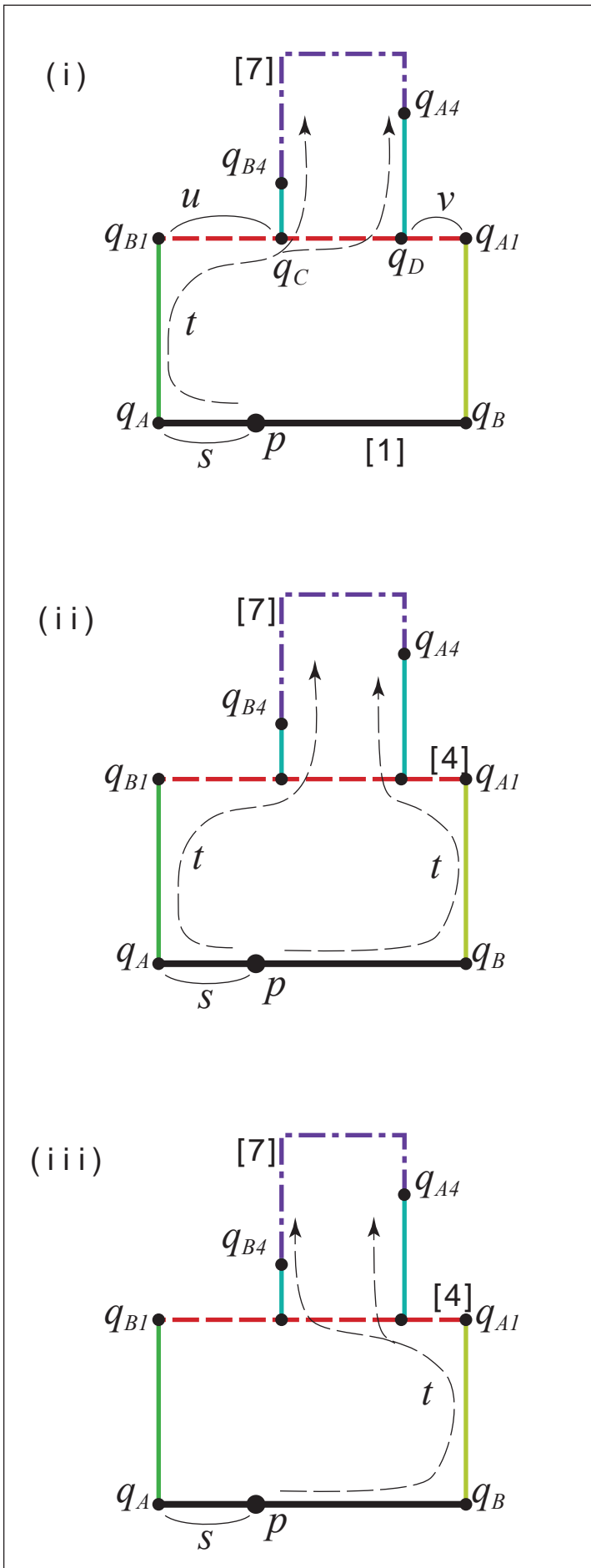
図 8: 軌跡リンク (グループ 4) の場合
