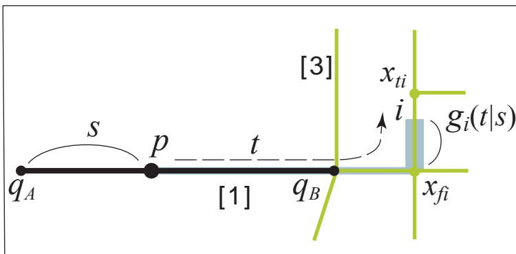
図 6: q_A からの最短経路が q_B を通るリンクの場合
